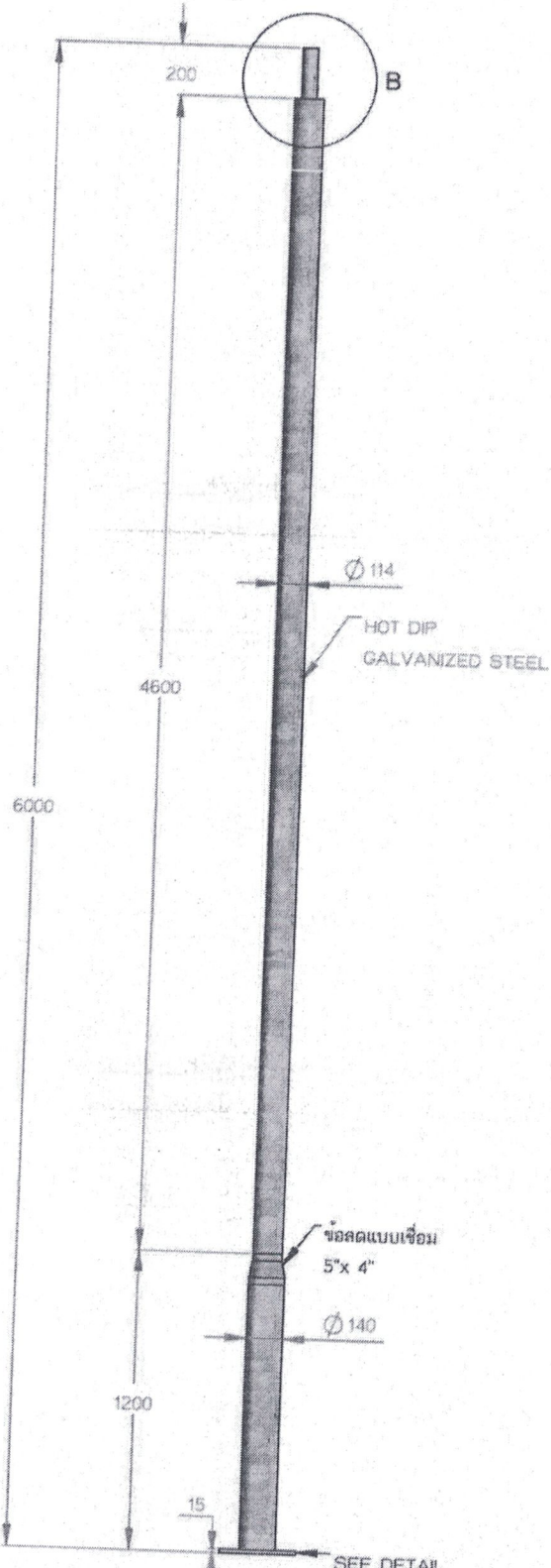
SEE DETAIL BASE PLATE HI-WC5-060:เสากลมสูง6เมตรขนาด5นิ้วลด4นิ้ว SCALE 1 : 28
